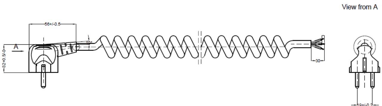
Spiralkabel
