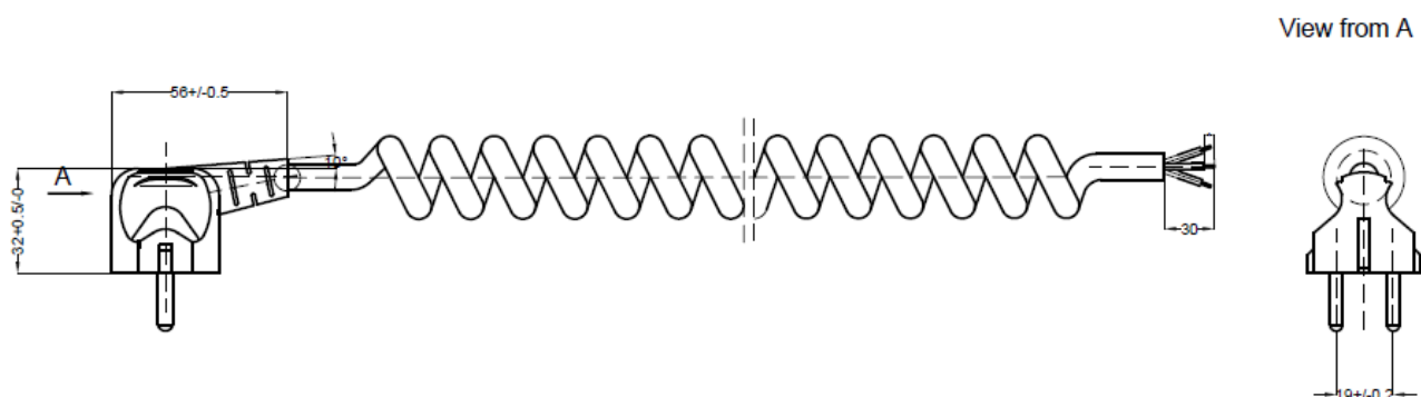
Spiralkabel
